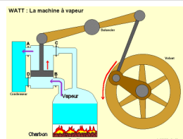
Machine à vapeur de James Watt
